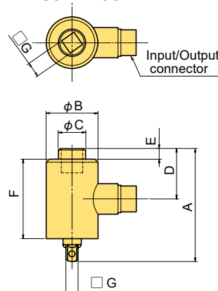
LTA-50 ~ -200NA
