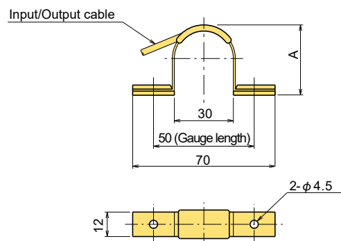
PI-2-50 / PI-5-50
