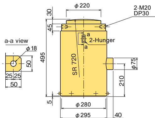
CLP-10MNB
