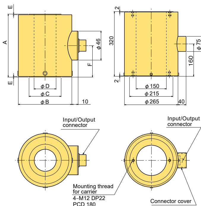
CLC-50KNA~ 3MNA
