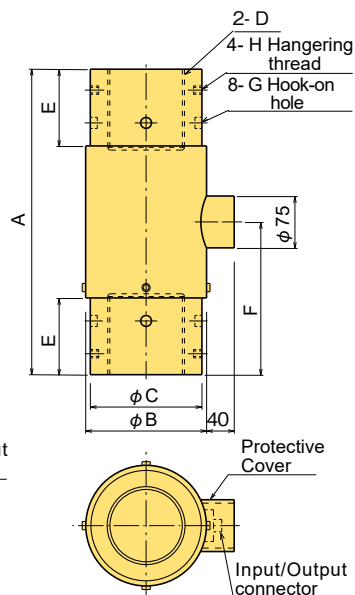
TCLP-1 ~ 2MNB
