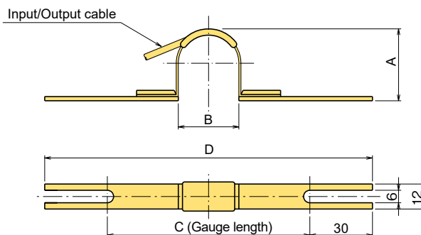
PI-2 / PI-5
