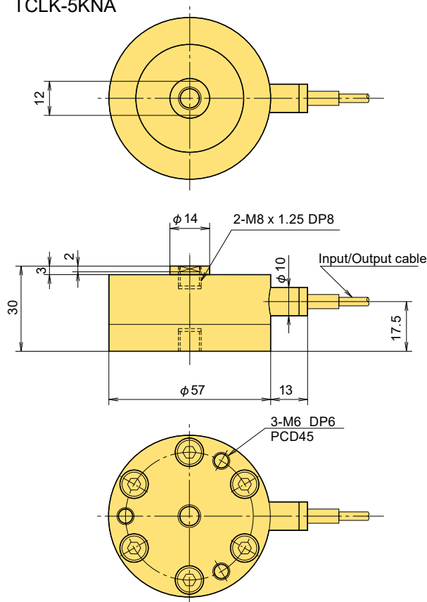
TCLK-5KNA
