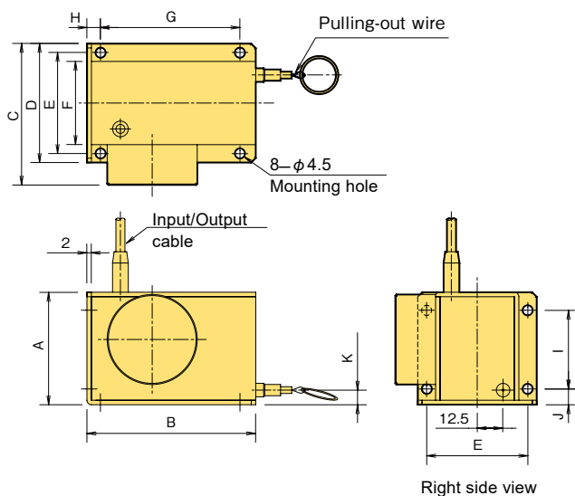
DP-500G/-1000G/-2000G
